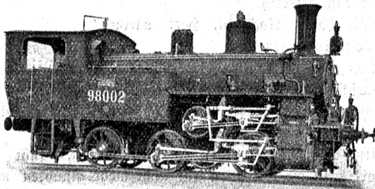
Lokomotive der Strecke Paola-Cosenza (Italien). Zwei getrennte Triebwerke für Adhäsions- und Zahnradbetrieb. Das Zahnrad ist deutlich sichtbar.
