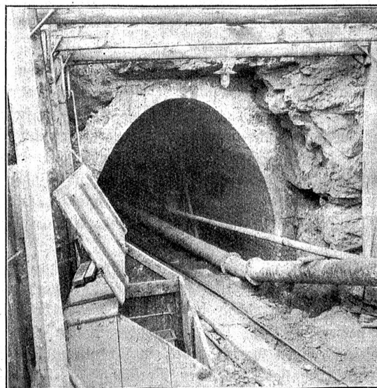
Sulgenbach-Stollen. Stollenportal Nordseite, fertig ausgemauert mit Ausnahme der Sohle. Rechts die Röhren für die Ventilatoren und die Preßluftleitung (3. Juni 1922).
