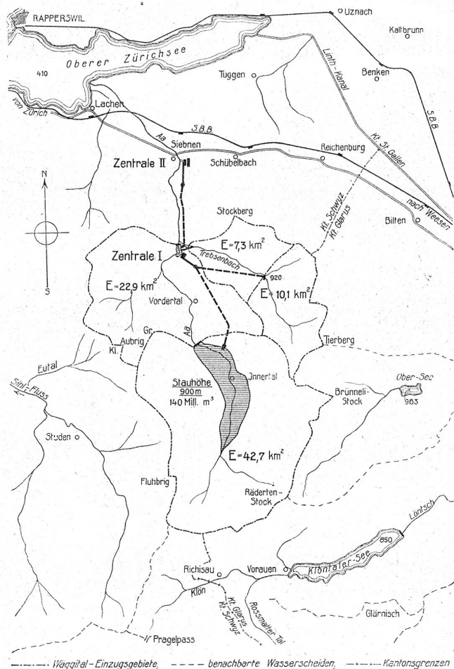
Das Wäggitalwerk. Klischee „Schweiz. Bauztg.“ Die Einzugsgebiete des Kraftwerks Wäggital. — 1:200,000.
