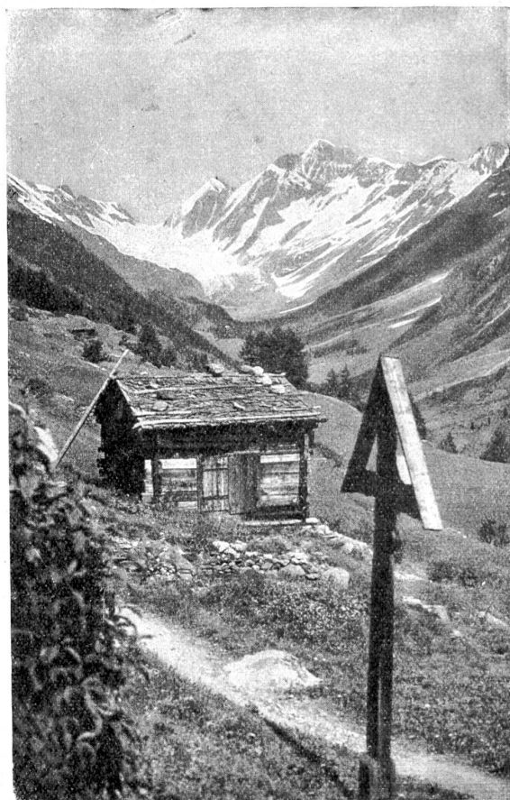
Oberes Löschental. Blick gegen die Löschentalücke.
