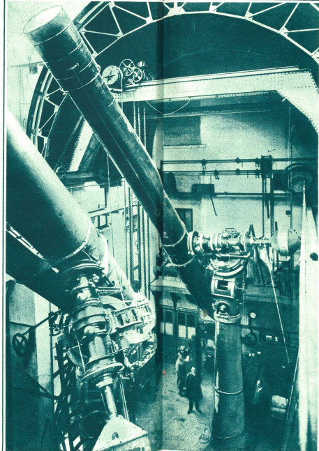
Ein Riesenferrohr auf dem Montagefeld der berühmten Zeiß-Werke in Jena, bestimmt für die Spitzweite in Belgrad.
