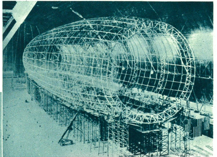
Das Gerippe des künftigen amerikanischen Luftriesen „7 R S — 4“, der gegenwärtig in der Bauhalle von Akron (Ohio) montiert wird. Mit einer Länge von über 260 Meter wird „7 R S — 4“ das größte Luftschiff der Welt sein.
