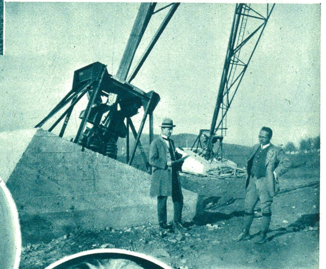
Unten: Verankerung und Isolierung der Turmpfeiler. Rechts außen der Konstrukteur der Antennentürme, Ing. Dick, von der Firma Bell in Kriens.
