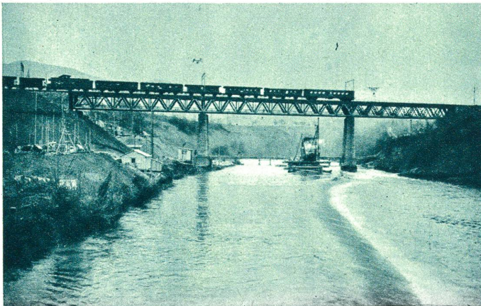
Der Bau des Limmatwerkes Wettingen. Photo E. A. Meili, Zürich.
