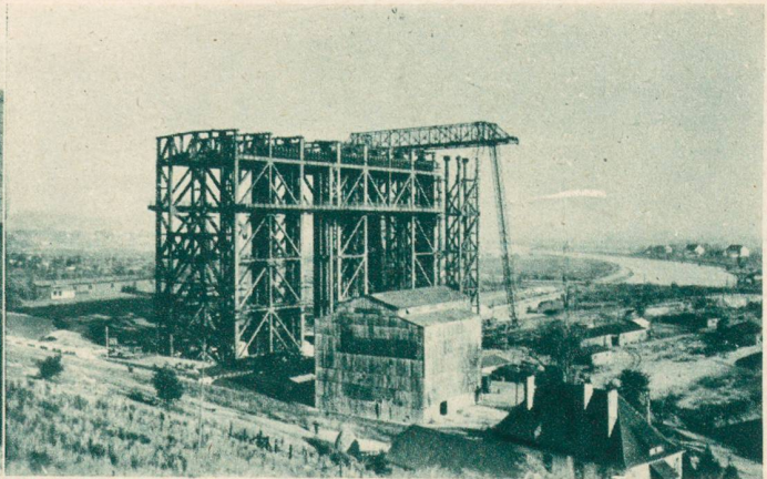
Ein riesiges Schiffshebewerk in Niederfinow (Deutschland), um Schiffe von einem Kanal in einen höher gelegenen zu heben. Atlantic-Photo.
