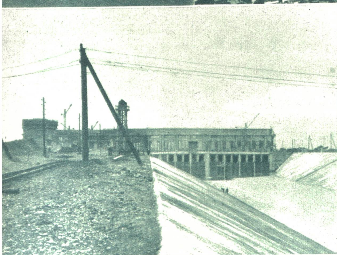
Das Großkraftwerk Kembs. Blick in die riesige Turbinenhalle. Im Mittelgrund wird eine der 33,000 P. S. Turbinen montiert und dann in die davor befindliche Kammer eingelassen. Unten: Der Oberwasserkanal beginnt sich mit Grundwasser des kleinern zu füllen, da derselbe nun nicht mehr abgepumpt wird.
