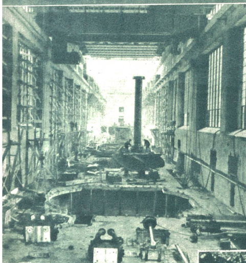
Das Großkraftwerk Kembs. Blick in die riesige Turbinenhalle. Im Mittelgrund wird eine der 33,000 P. S. Turbinen montiert und dann in die davor befindliche Kammer eingelassen. Unten: Der Oberwasserkanal beginnt sich mit Grundwasser des kleinern zu füllen, da derselbe nun nicht mehr abgepumpt wird.
