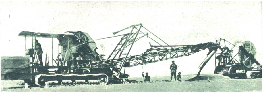
Die Maschine macht Menschen überflüssig. Eine riesige Kabellegemaschine, die den Graben gräbt, das Kabel legt und den Graben wieder zudeckt. Bedienung: 4 Arbeiter, statt vorher 45. Phot. International Graphic.
