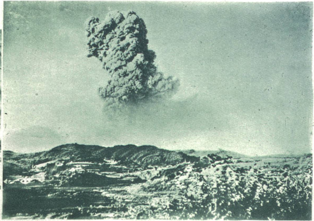
Eine riesige Eruption des japanischen Vulkans Asama, durch die zahlreiche Dörfer in Brand gesteckt und vernichtet wurden. Die in Japan so häufigen Erdbeben stehen jedenfalls in Zusammenhang mit der Tätigkeit der zahlreichen noch aktiven Vulkane. Atlantic Photo.
