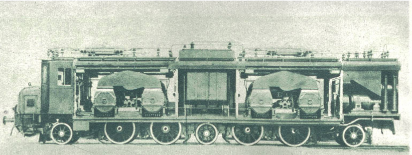
Die größte Lokomotive der Welt — 8800 PS! Die Maschinenfabrik Oerlikon lieferte kürzlich den S. B. B. die für die Gotthardbahn bestimmte Maschine ab. Das Bild zeigt die Innenkonstruktion der einen Hälfte der Riesenmaschine. Cop. Photopress Zürich.
