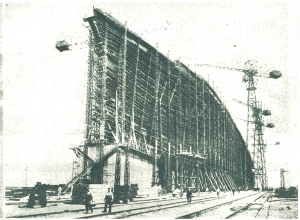
Der größte Ozeandampfer der Welt wird in Frankreich auf den Werften von St. Nazaire gebaut. Es ist dies die »Super-Ile-de-France«, welche der größte und schnellste Dampfer der Welt werden soll. Unser Bild zeigt den gegenwärtigen Stand der Bauarbeiten an diesem Schiff. Associated Press.
