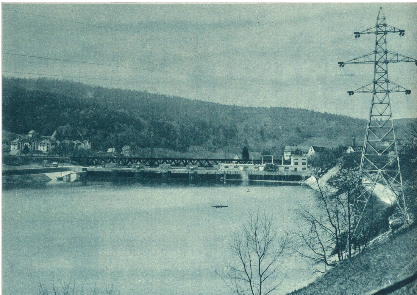
Zur Vollendung des Limmatkraftwerkes bei Wettingen. Blick auf den Stausee mit dem Wehr und dem Turbinenhaus. Phot. A. Krenn, Zürich.
