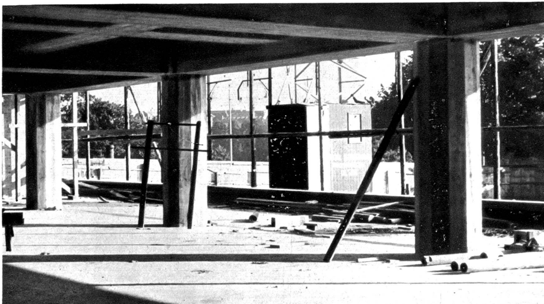
Durchblick beim Parterrege-schoss. Diese Zwölfecksäulen tragen das ganze Gebäude. Sehr schwierig war die Ausführung der Fundationen auf diesem Baugelände
