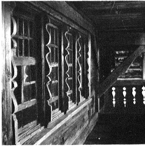
Abb. 2. Gadenfenster an einem Hause bei Köniz (Bachtelen) aus dem Jahre 1718. Beste Zimmermannsarbeit.
