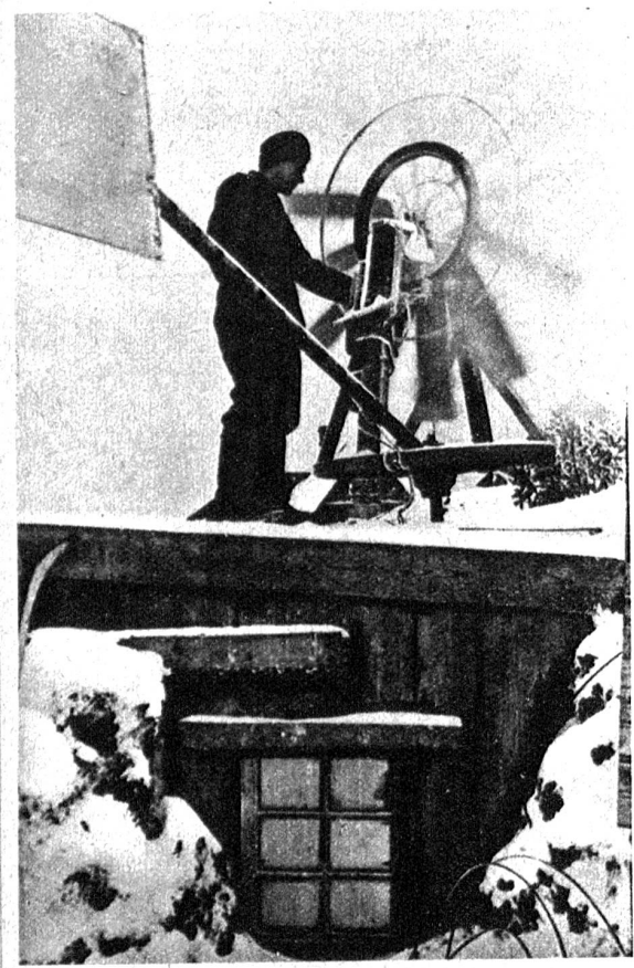
Eine Bunkerbesatzung an der nördlichen Front vor Leningrad hat sich den kalten Ostwind zunutze gemacht, indem sie mit einem Windrad, 2 Veloreifen und 2 Dynamos ein kleines Elektrizitätswerk schuf, das neben Licht auch etwas Wärme spendet
