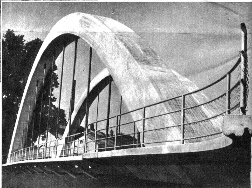
In Emmenbrücke bei Luzern haben die L. von Roll'schen Eisenwerke eine Werkbrücke gebaut, die in ihrer Konstruktion in Europa einmalig ist. Die Betonbrücke, die den Fluss schräg schneidet, weist durch die besondere Form der Aufhängung das Tragmoment in der Diagonale auf (Zens.-Nr. 7450 BRB 3. 10. 39.,
