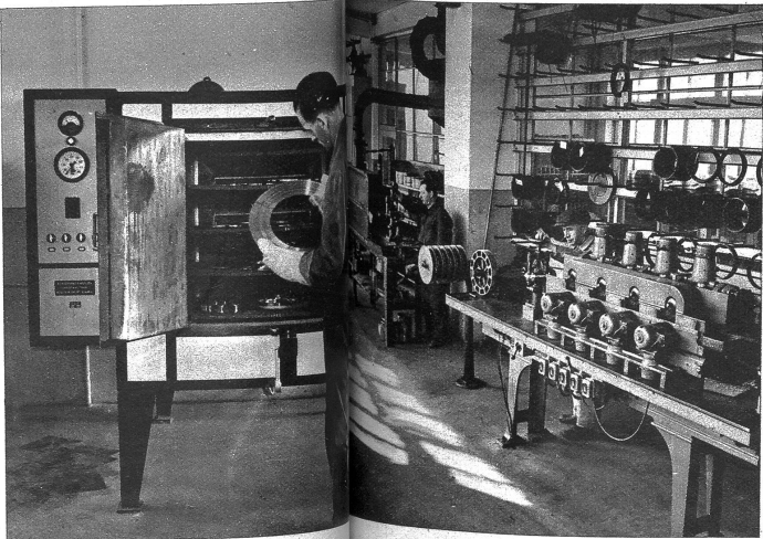
Elektrischer Warmluftofen zum Anlassen von Uhrenfedernbändern bei einer Temperatur von zirka 500°C. Links: Die Kontrolle auf Härte und Elastizität im Labor. Rechts: Ansicht des Arbeitsraumes, in welchem die Uhrenfedernbänder zu Spiralen gewickelt werden.
