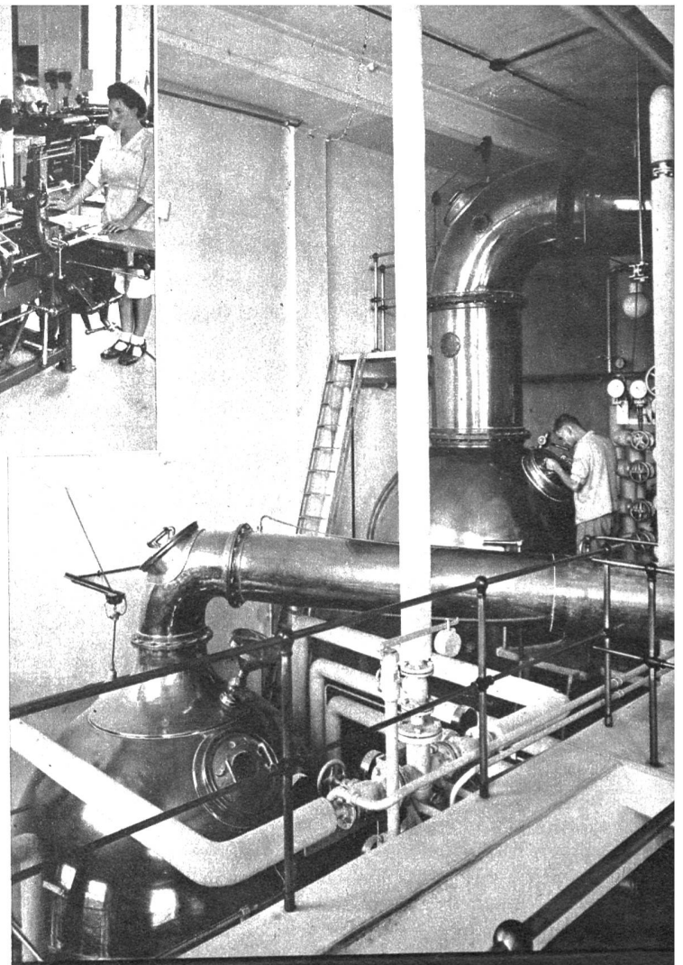
Vakuum-Eindampfapparat
