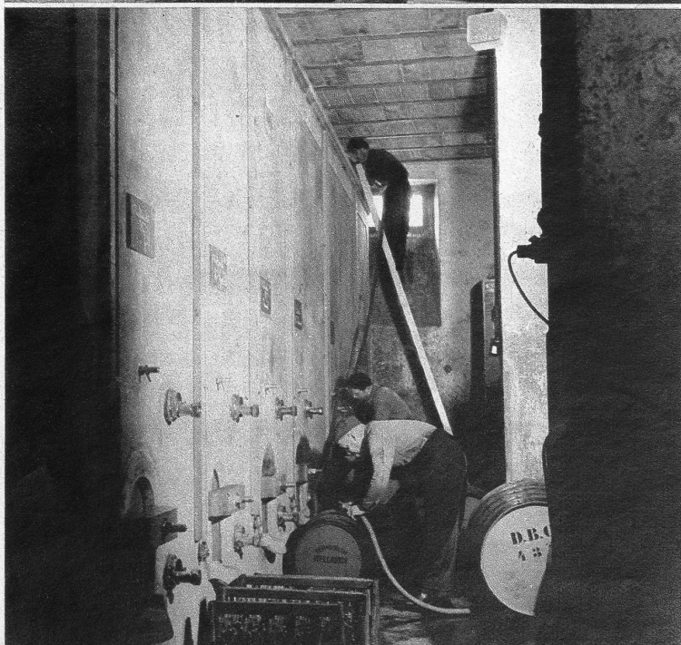
Links: Keller mit Borsari-fässern, welche je 10 000 l zu fassen vermögen
