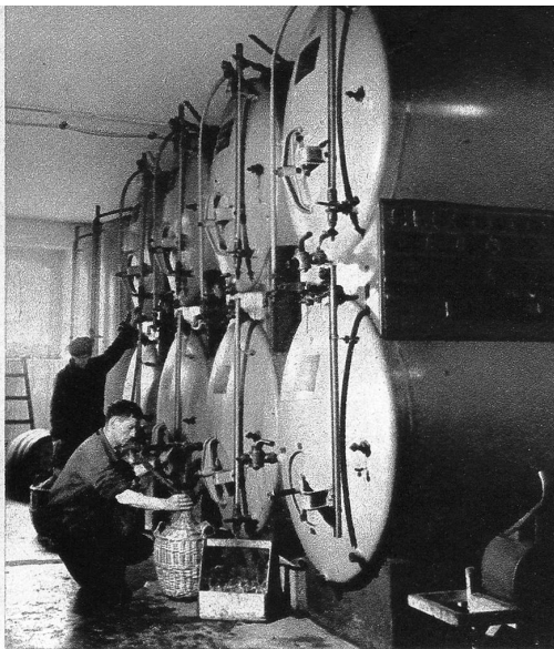
Tankanlage für Qualitätsspirituosen mit 30 000 l Fassungsvermögen
