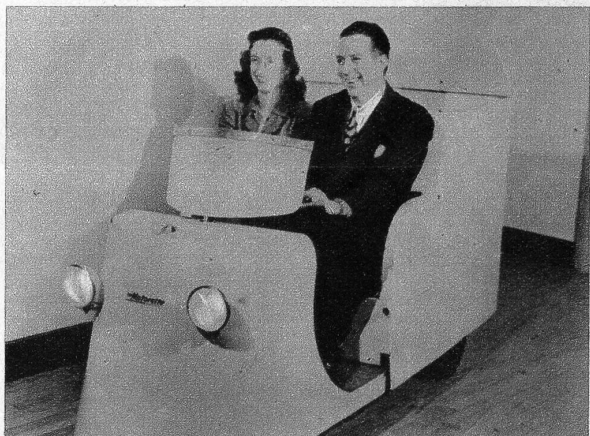
In Neuyork erblickte die «Motorette» das Licht der Welt. Das dreirädrige Fahrzeug ist vollständig aus Aluminium hergestellt und besitzt einen Zweizylinder-Motor, automatische Kupplung und Schaltung sowie einen elektrischen Starter. Die «Motorette» verbraucht auf 130 Kilometer 4 Liter Benzin.
