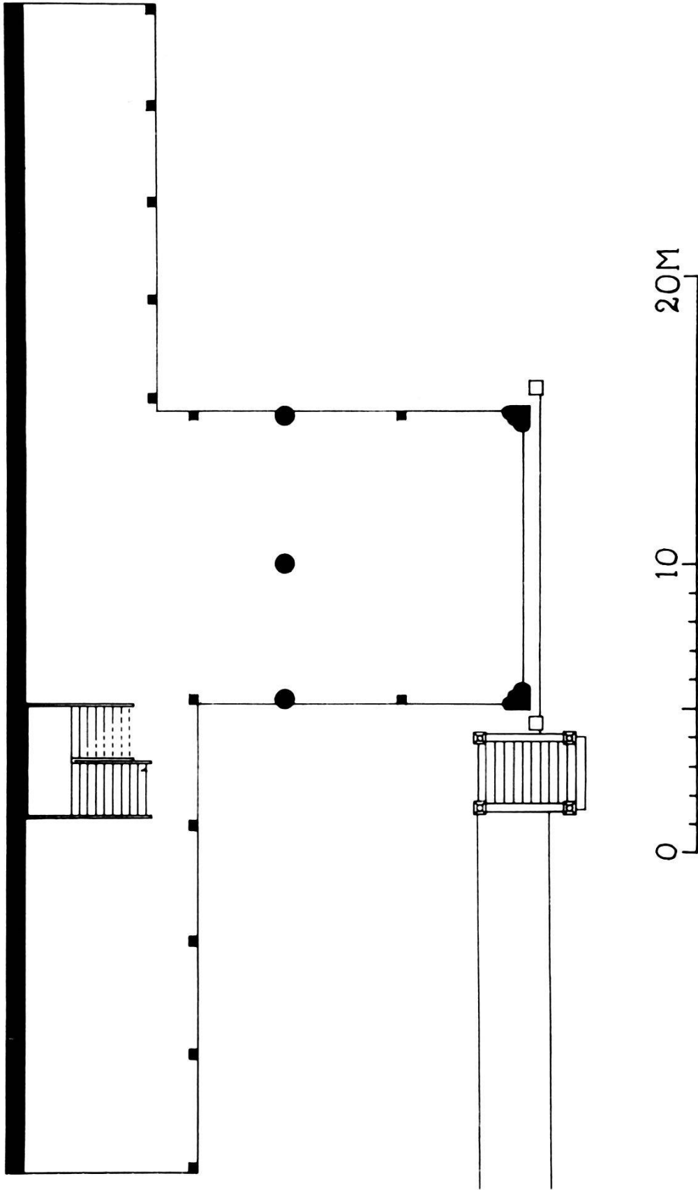
Abb. 7. Grundriss des Stachelschützenhauses 1729. Der gegen das Spalenter hin längs der Stadtmauer neu errichtete Südflügel wurde für den physikalischen Experimentaltunnterricht gebaut. Das zunächst offene Erdgeschoss liess man 1732 zu einer Wohnung für den Schützenknecht ausbauen. (Bild. Bürgerhaus Mappe 17, Nr. 6)
