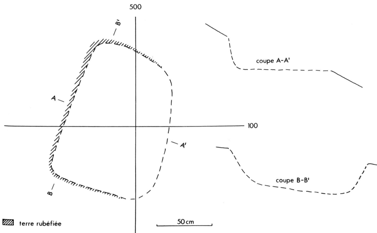
Fig.93 Gumefens . Relevé de la fosse (1:50)
