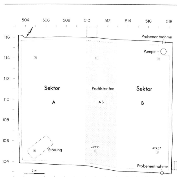
Abb. 21 Muntelier/Fischergässli. Sektorenplan
