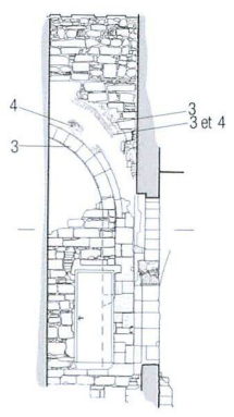
Mur nord/Nordmauer
