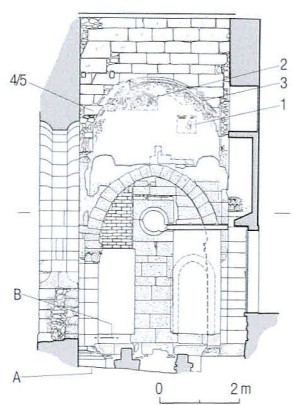
Mur est/Ostmauer
