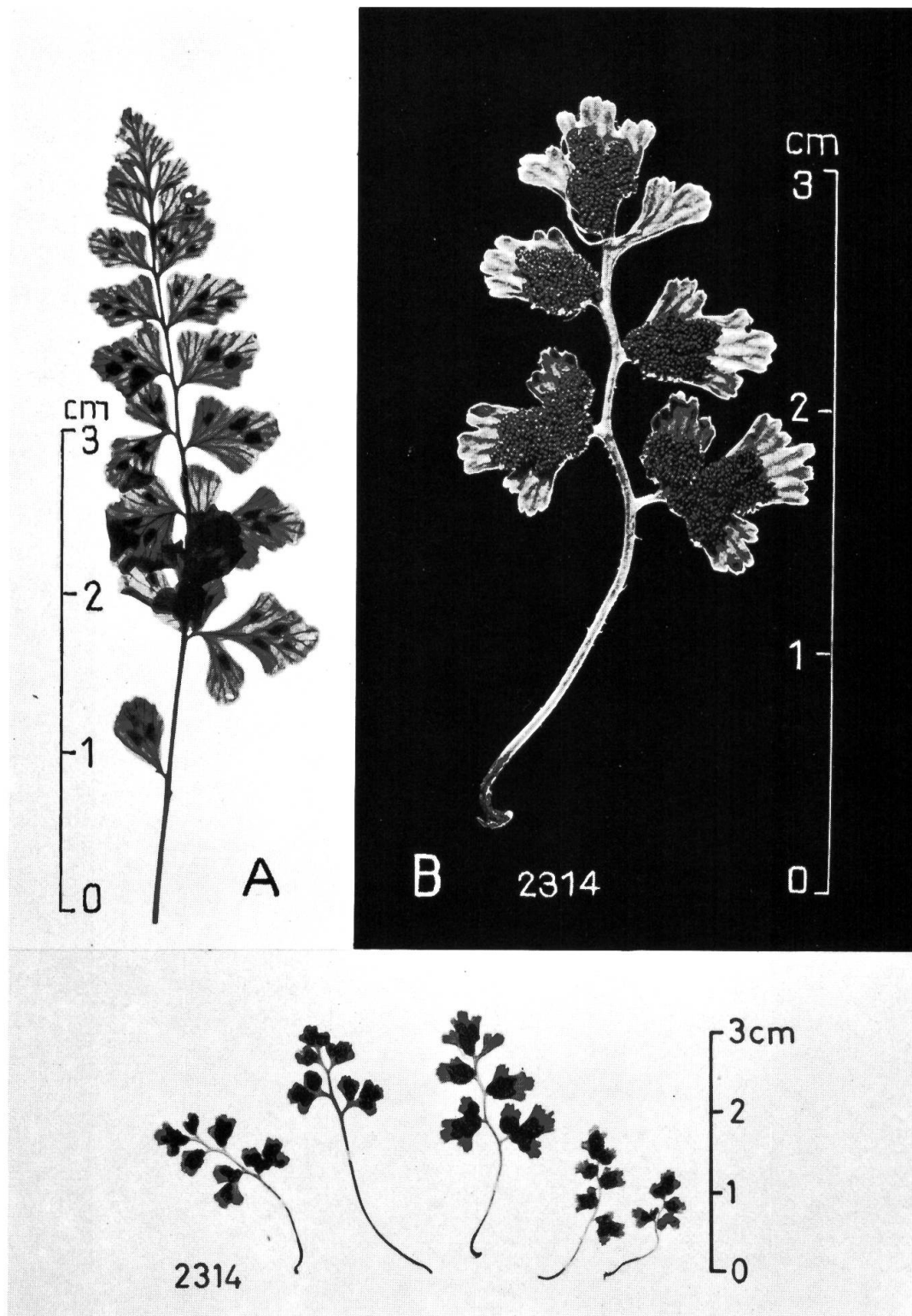
Fig. 2. — Einzelwedel: A, Asplenium x reuteri im Durchlicht, 2 x vergrössert, zeigt Nervatur; B, A. haussknechtii (TR 2314), überreif, vom locus classicus des A. x reuteri , im Durchlicht, 3 x vergrössert; C, A. haussknechtii (TR 2314), 5 Wedel in natürlicher Grösse.
