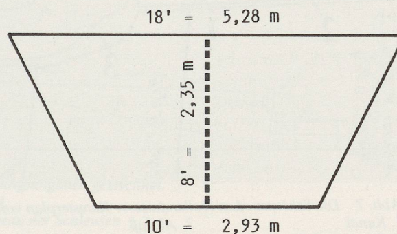
Abb. 6 Theoretisches Profil (Schnittzeichnung) des Kanals.
