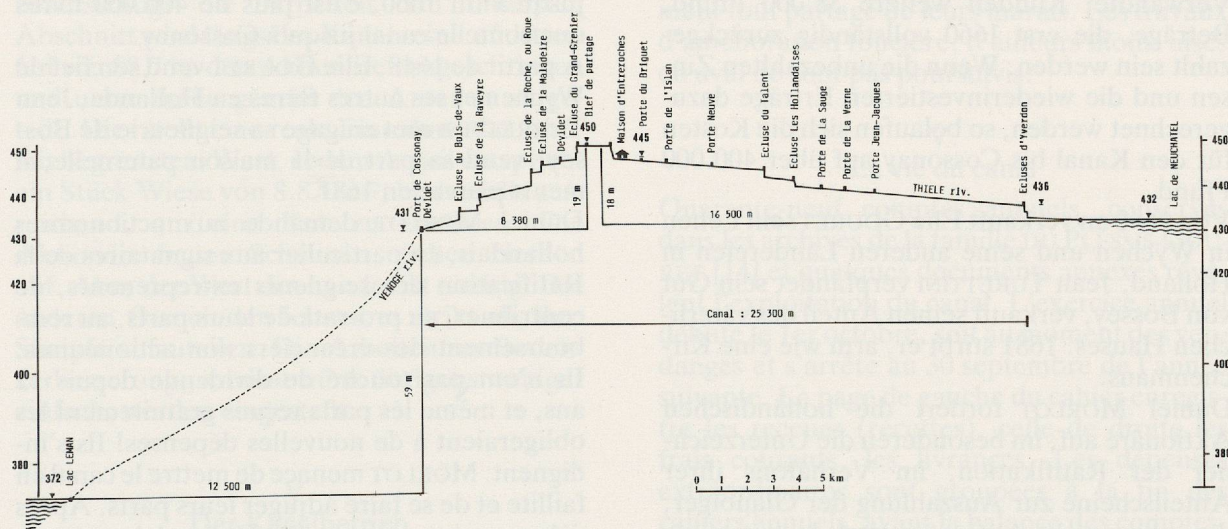
Abb. 10 Theoretisches Profil des Kanales von Entreraches. Fig. 10 Profil théorique du canal d'Entreraches.
