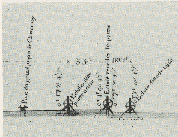
Abb. 9 Detail der Radschleusen in der Nähe der »Six Portes«, auf der Kopie eines im Jahre 1640 aufgenommenen Profils (Waadtländer Kantonsarchiv).
