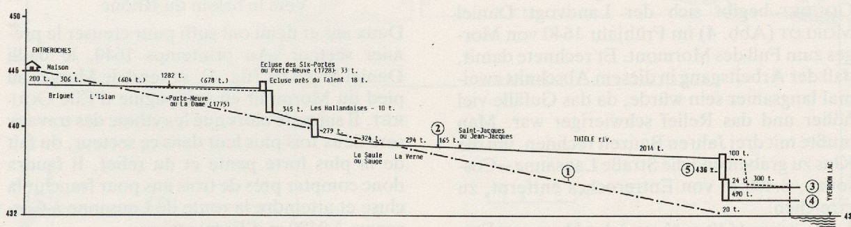
Abb. 8a Profil des Kanals von Entreroches, nach alten Vermessungsangaben gezeichnet.
