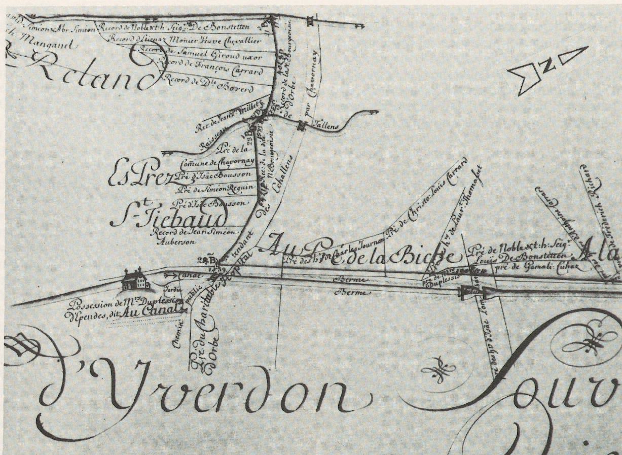
Abb. 13b Der Hafen von Talan, der Kanal, seine Bermen und die Kammerschleuse »les Hollandaises«. Plan aus dem Jahre 1756 (Waadtländer Kantonsarchive).
