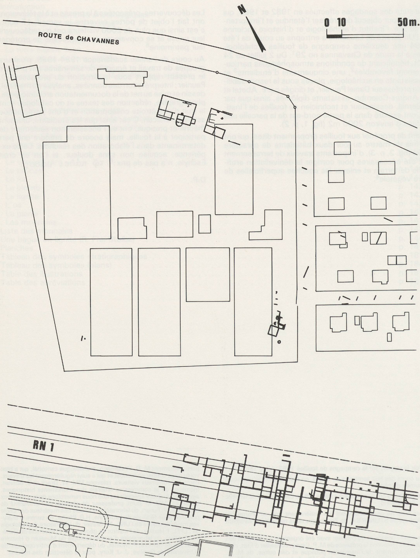
Fig. 1. Situation générale.
