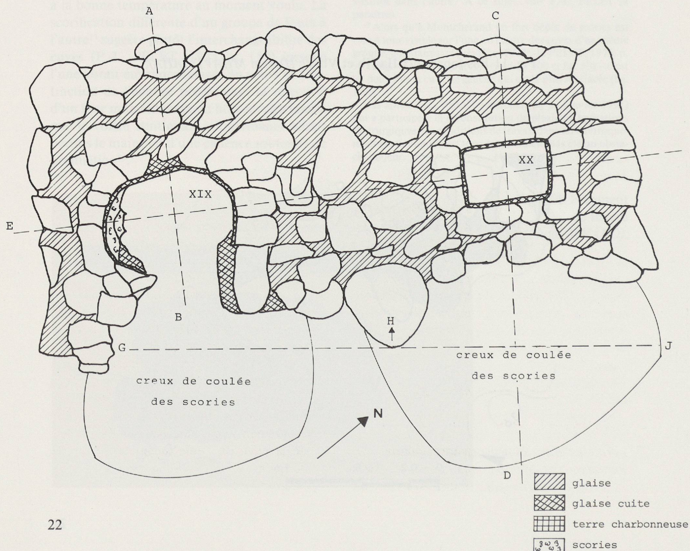
Fig. 12 Fours doubles sur le site de Bellaïres; fours III et IV de Bellaïres I et fours XIX et XX de Bellaïres III, tirés de P.-L. PELET (1973, pp. 95 et 100, fig. 46A et 50).
