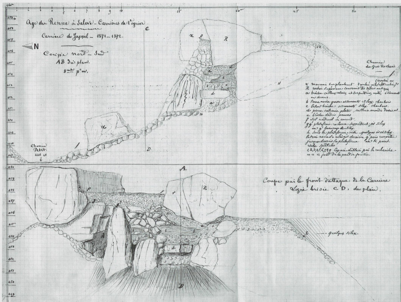
Fig. 69 Coupe manuscrite de l'abri Gosse dans la carrière Jappel, par A. Rochat. Datée probablement de 1872. Légende du cartouche: « Alpha: morceau surplombant, tombé en octobre ou septembre 71. R: rocher supérieur couvrait les débris antiques. a: brèche caillouteuse calcaire et serpentine mêlés, ossements en dessous. b: terre noire grasse ossements silex charbons. c: béton brèche ossement silex charbons. d: pierre calcaire plate, cailloux arrondis dessus os. e: brèche débris pauvres. f: sol naturel en amont. g: plateforme rocheuse supportant os et silex en g' beaucoup de silex. h: sous la plateforme vidé quelques os et silex. La terre noire se relevait derrière g' pour remonter jusque dessus de la plateforme en K point riche spatules. 1, 2, 3, 4, 5, 6, 7, 8, 9, Espace déblaié par la recherche. 10, 11, 12 fond de la partie fouillée. »
