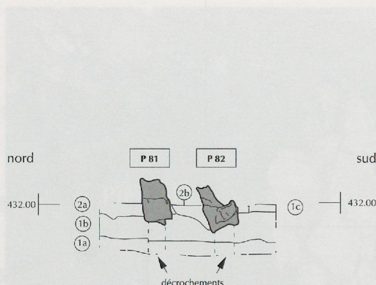
Fig. 88. Secteur sud, Philosophes 27, tronçon 6. Coupe nord-sud, vue est, en travers des poteaux ST 81 et 82 (situation fig. 79). Ech. 1:20.
