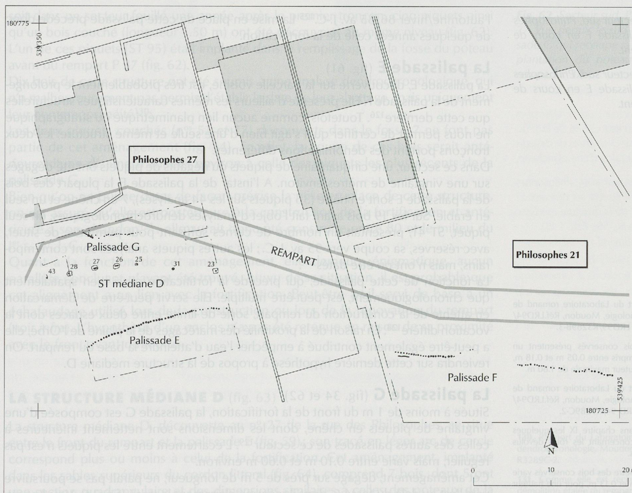
Fig. 59. Secteur sud. Plan des vestiges découverts devant le rempart.
