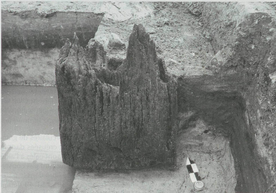
Fig. 71. Secteur sud, Philosophes 21, tronçon 5. Poteau arrière P 106. La base de ce bois, dont la hauteur originelle est estimée à près de 6 m, est parfaitement conservée en raison de la proximité de la nappe phréatique.
