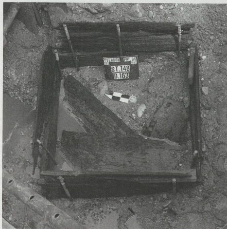
Fig. 136. Secteur oriental, Philosophes 7. Le puits ST 148 en cours de dégagement.
