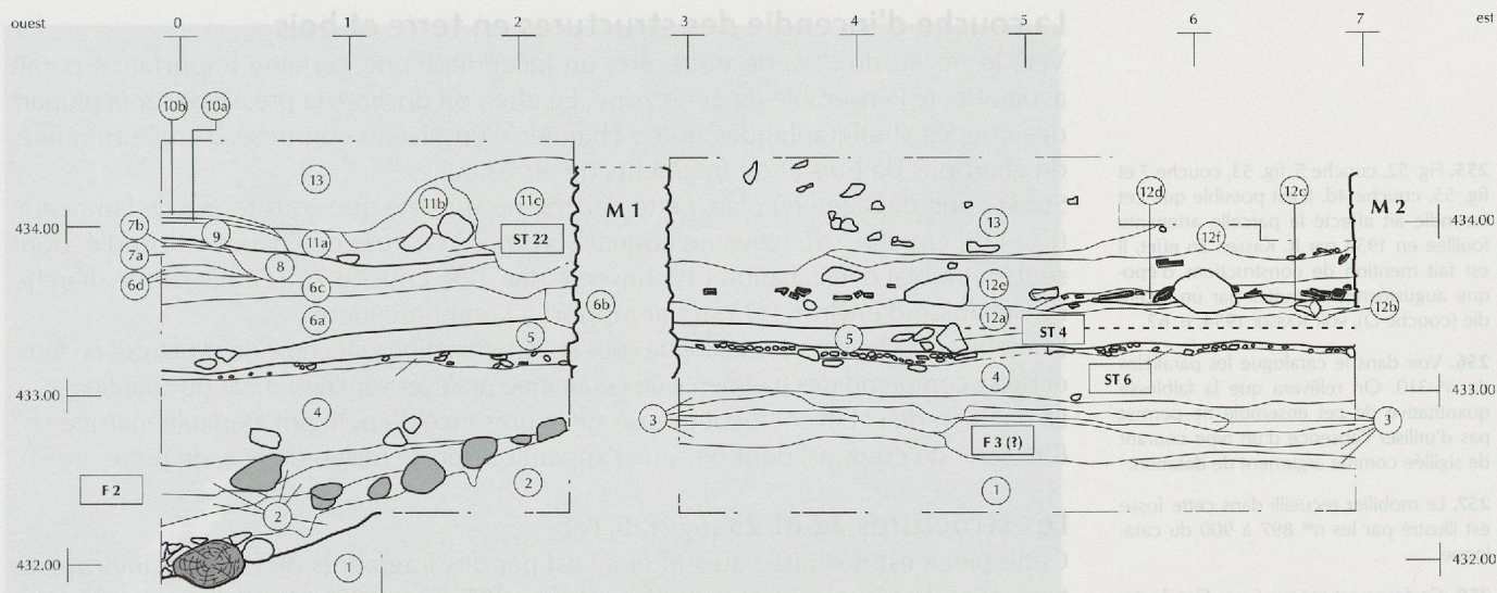
Fig. 129. Secteur oriental, Philosophes 13. Coupe stratigraphique ouest-est, vue nord, à travers la cave et à l'ouest de M1 (situation fig. 127).
