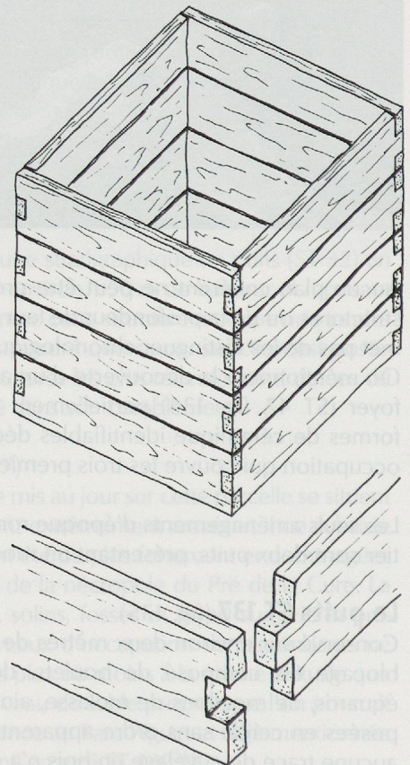
Fig. 137. Reconstitution et détail du mode d'assemblage des planches du cuvelage du puits ST 148. Dessin D. Widmer.
