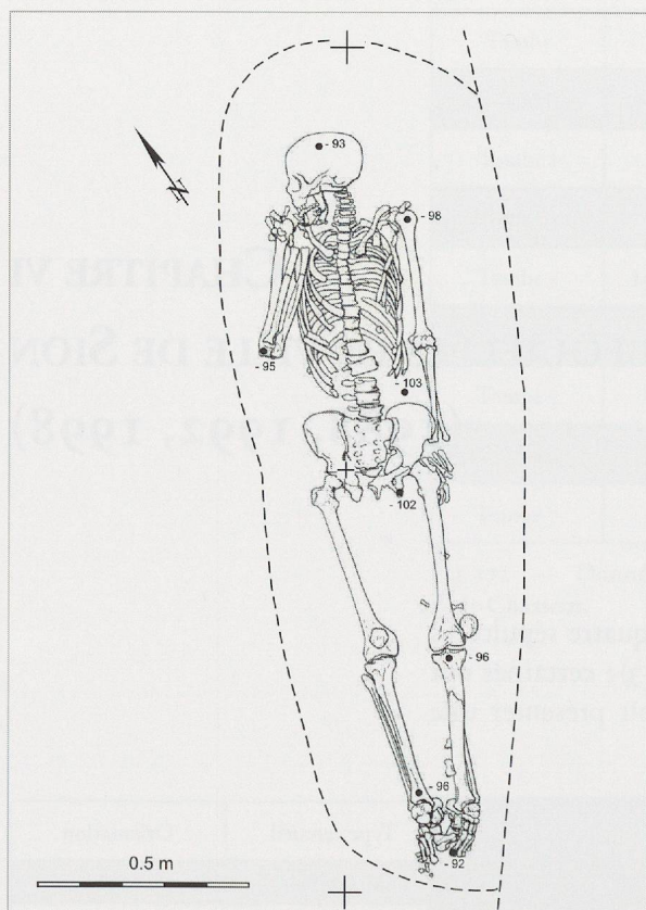
Fig. 176 — « Ancienne Placette ». Plan de la tombe 5 au niveau du squelette. Ech. : 1/20.
