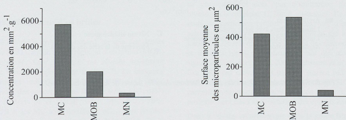
Fig. 4: Quantification de la présence des microrestes biologiques et minéraux noirs au cours du protocole d'extraction palynologique.
