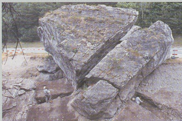
Fig. 29 — Möderstein. Rocher vu depuis le nord.
