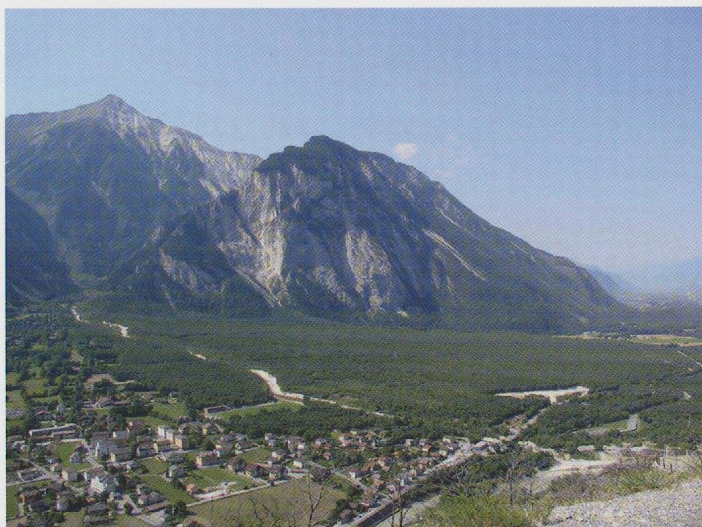
Fig. 56 — Cône et torrent de l'Ilgraben. Au premier plan, le village de Susten ; à droite, la clairière du bois de Finges. Vue depuis les hauteurs du bourg de Leuk.
