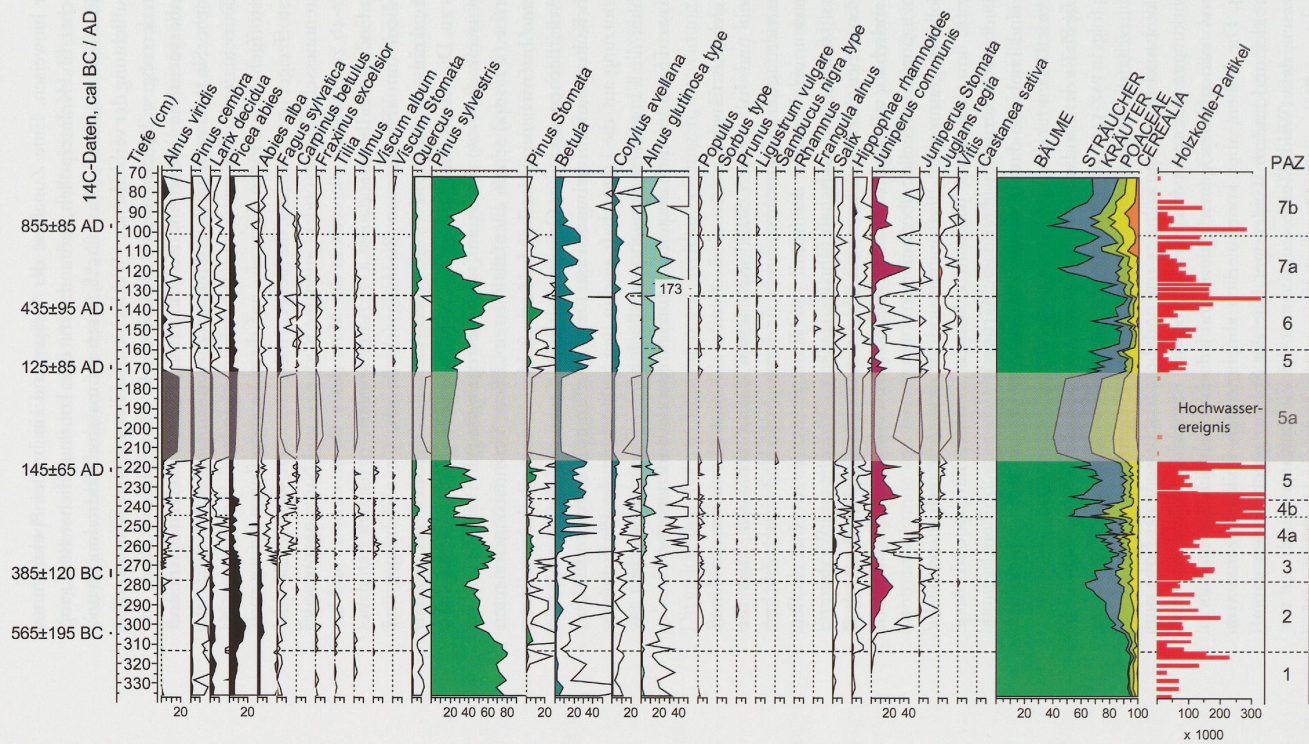
Fig. 368 — Pollendiagramm des Profils Pfafforetsee PF07_1/2 mit den Prozentwerten der wichtigsten Bäume und Sträucher. Kurven mit niedrigen Werten sind 10-fach überhöht dargestellt (schwarze Linie). Die mikroskopische Holzkohle ist als Anzahl Partikel pro cm 3 Sediment angegeben.
