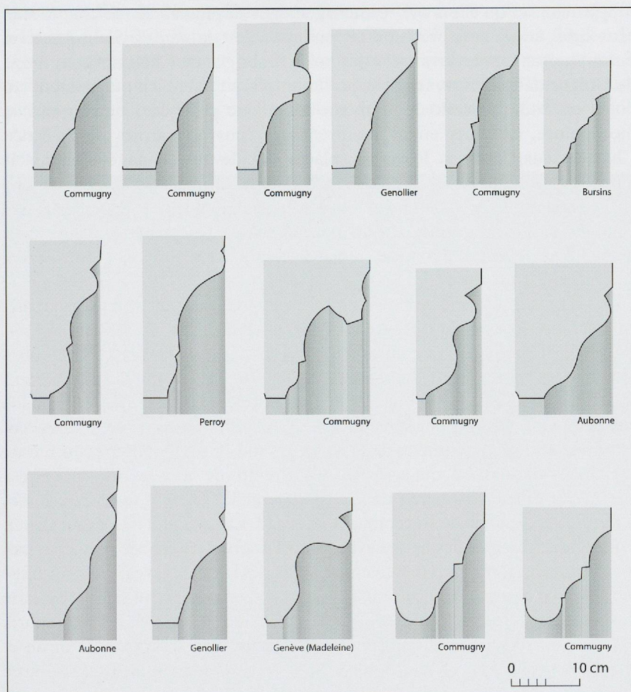
Fig. 329. L'église Saint-Christophe de Commugny. Tableau de profils d'ogives relevés sur la Côte vaudoise (relevés MG et dessin de Marion Berti, Service cantonal d'archéologie, Genève). Voir aussi fig. 173 et 306 (Morges).
