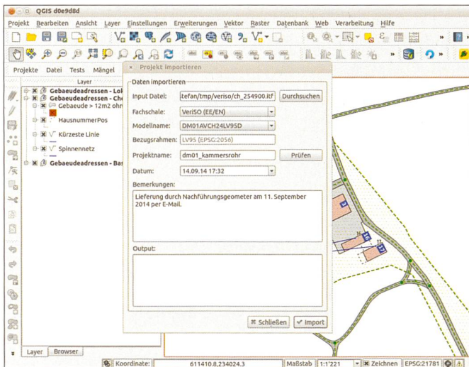
Abb. 1: Importdialog mit Auswahl der Fachschale, des Datenmodells und des Bezugsrahmens
