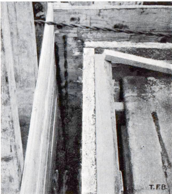
Abb. 2 Isolierung einer Eisenbetonwand mit einer 5 cm versteinerten Holzwoolplatte, die ebenfalls als Innenschalung dient.
