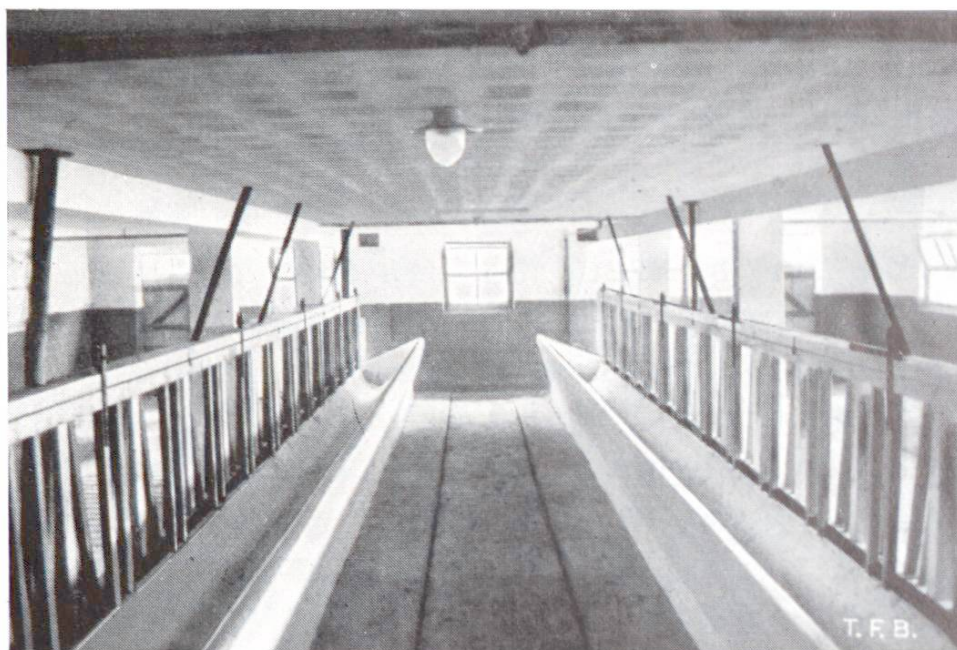
Fig. 6. Hallenfall mit armerter Hohlkörperdecke und armerter Stützen. Die massive Bauart ist wirtschaftlich, hygienisch und feuersicher.
