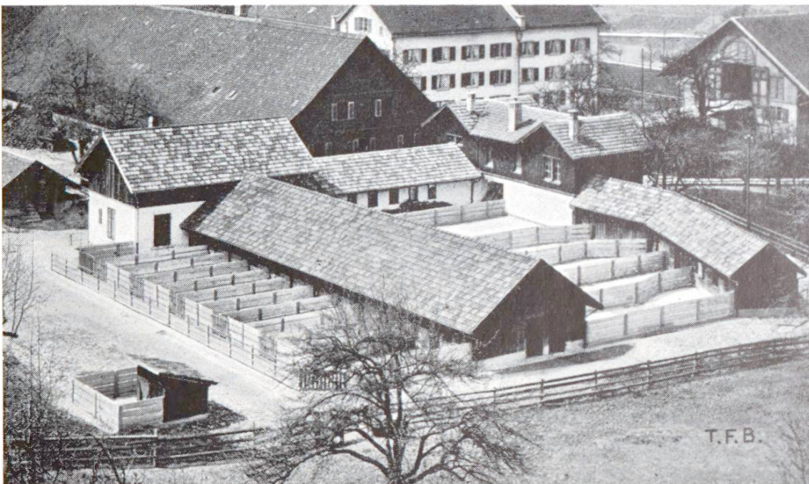
Fig. 5. Schweinställe der Landwirtschaftlichen Schule Strickhof, Zürich. Betonierte Auslaufplätze, Zäune aus Betonpfosten und Betonbrettern.
