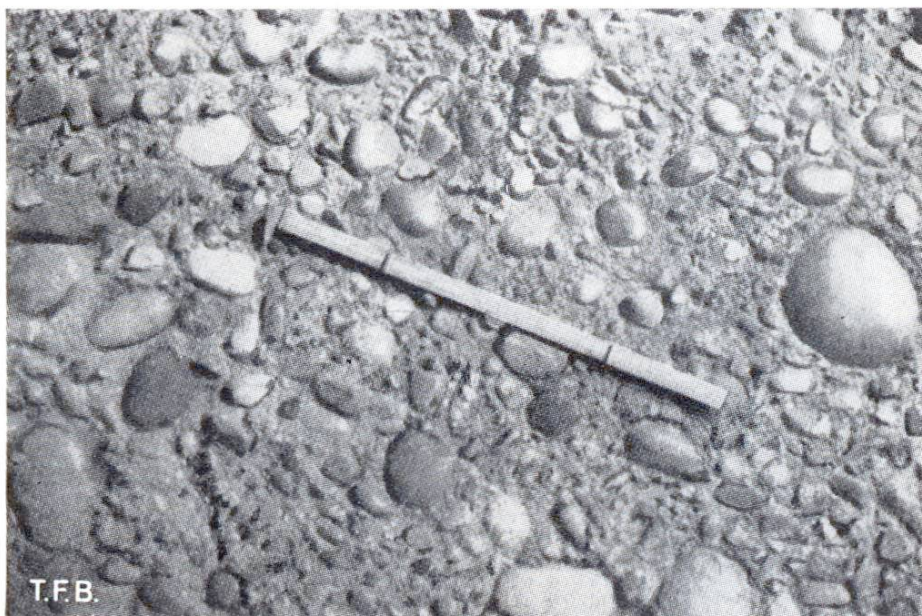
Abb. 11 Beton nach Aufrauung
