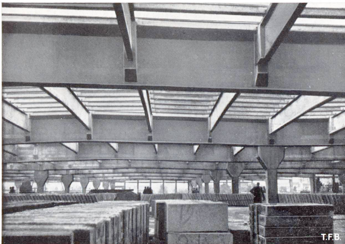
Abb. 8 Baumwollfabrik Gand (Belgien), Innenansicht mit Bindern, Pfetten und Sparren aus vorgespanntem Beton, System Magnel. Im Gegensatz zu Eisenbeton und wie bei Stahlprofilen wirkt hier der Untergurt statisch mit
