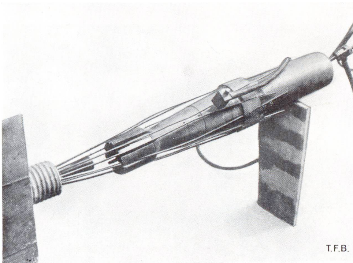
Abb. 1 Spannvorrichtung nach Freyssinet, hydraulische Presse zum Ziehen des konisch erweiterten Drahtbündels und zum Einpressen des Propfens (aus Ostenfeld: For-spaendt Beton Kopenhagen 1949)
