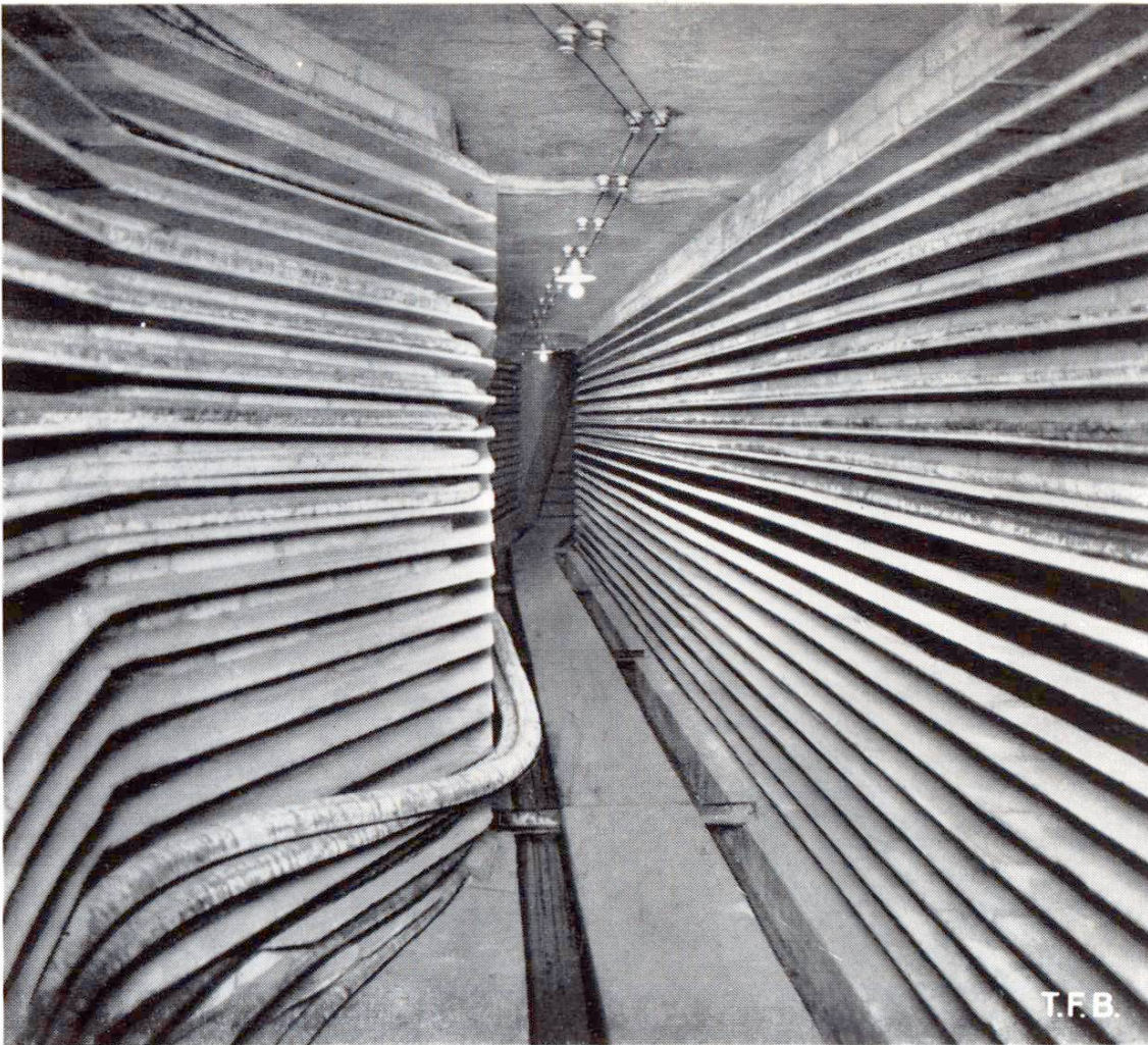
Abb. 7 Kabelgang in einer Transformatorenstation
