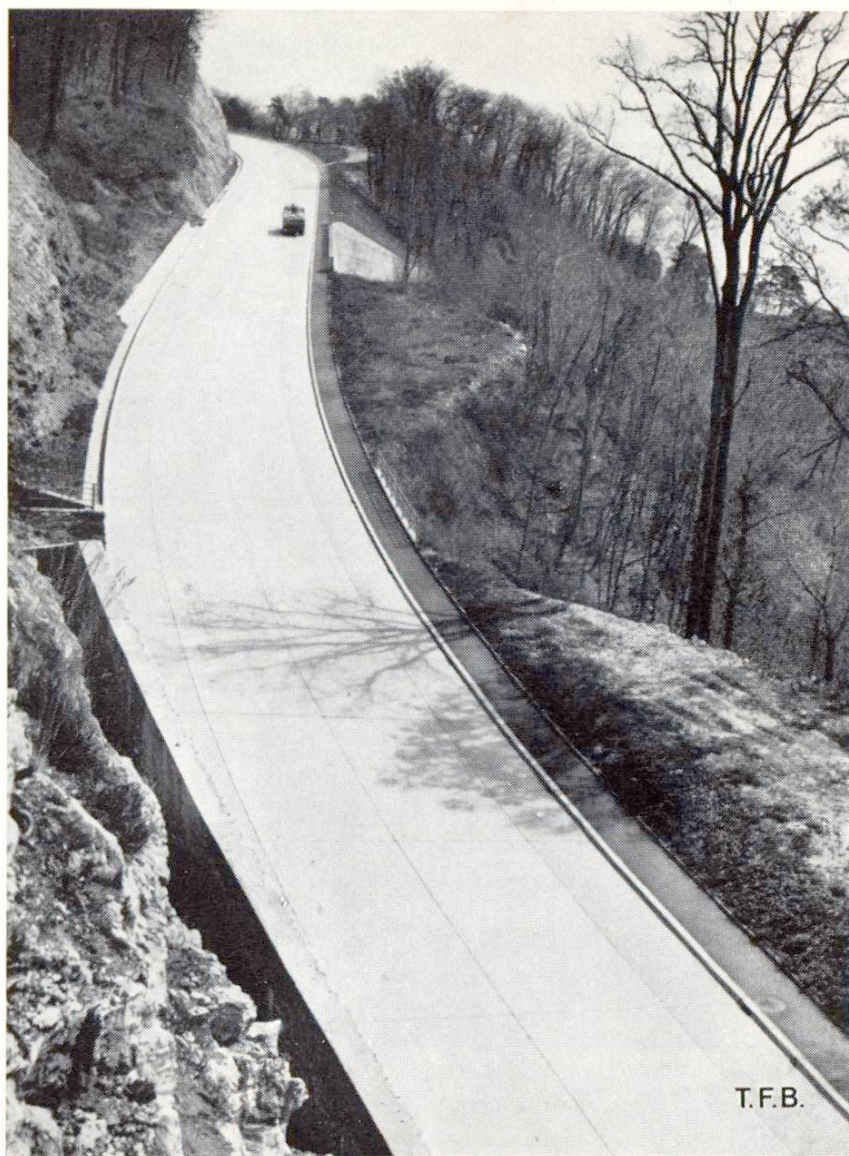
Abb. 12 Eindrückliche Streckenführung der neuen Betonstrasse bei Concise am Neuenburgersee. Helle Betonfahrbahn und rotgetönte Beton-Fahrradstreifen
