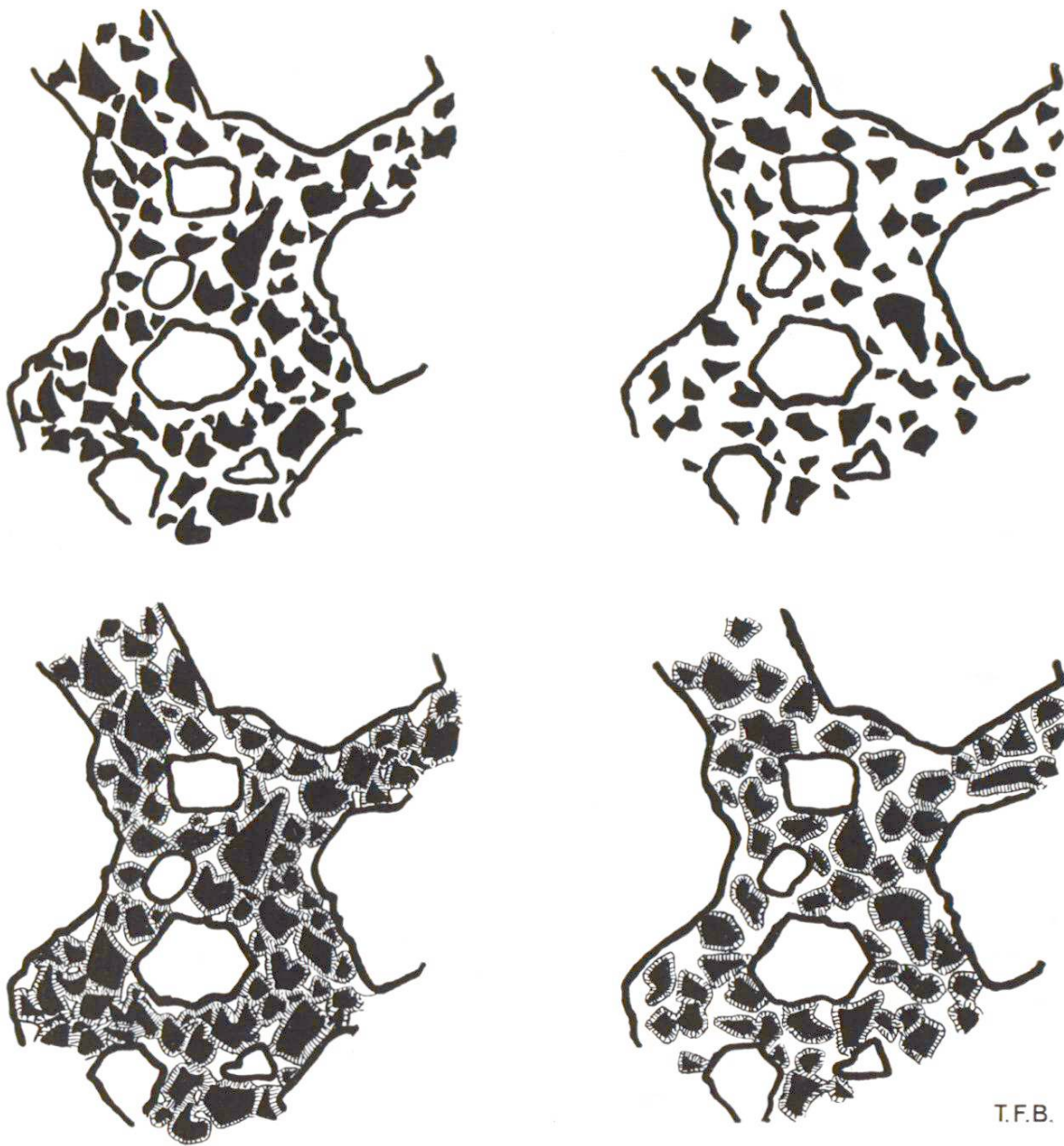
Abb. 3 Bildung von Kapillarporen im Cementleim eines Betons. Oben: frisch angemacht, unten: hydratisiert (erhärtet). Links: Wasser-Cement-Verhältnis ca. 0.5 — durch die Volumenvergrößerung sind die Kapillarporen in sich abgeschlossen worden. Rechts: bei einem Wasser-Cement-Verhältnis von über 0.7 wird trotz derselben Volumenvergrößerung der Festsubstanz keine geschlossene Porosität mehr erreicht.
