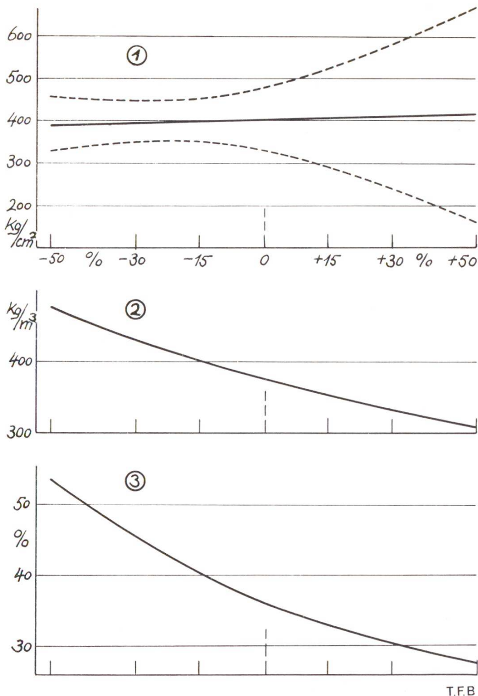
Abb. 2 Auswirkungen von Fehlern in der Kies-Zumessung von -50\% bis +50\% auf die Betondruckfestigkeit (1), die Cementdosierung (2) und den Sandgehalt des Zuschlags (3). Die gestrichelten Kurven in Diagramm (1) geben einen Streubereich der Betondruckfestigkeiten an, und zwar entfällt, gemäss der Wahrscheinlichkeitsrechnung, unter 370 Versuchen einer ausserhalb dieser Grenzen. Bemerkenswert ist, dass die Festigkeitsstreuung mit zunehmenden groben Kornanteilen beträchtlich grösser wird (nach Vironnaud)
