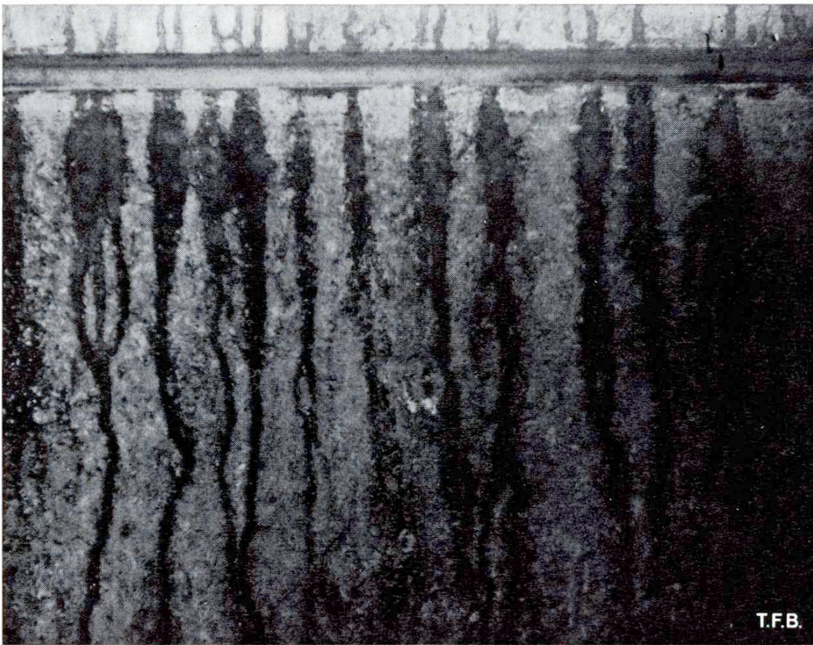
Abb. 8 Rasch fliessendes Niederschlagswasser kann eine frische Kalkausscheidung wieder auflösen.
