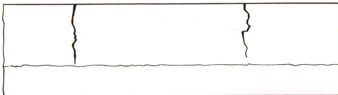
Abb.7 Ist die schwindende Schicht dick, so fällt der Risseabstand und die Rissweite relativ gross aus. Bei länglichen, balkenförmigen Bauteilen entstehen einzelne unverzweigte Risse senkrecht zur Längsachse.
