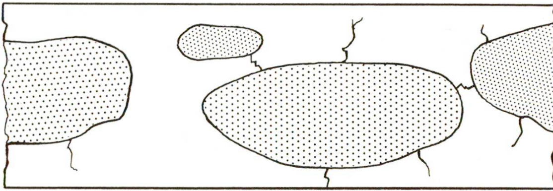
Abb.5 Interne Risse infolge Schwindzwängung im Bereich grösserer Zuschlagskörner. Wenn keine Risse entstehen, so sind Zugspannungen vorhanden, die gegebenenfalls das Resultat der Festigkeitsprüfung verfälschen, d. h. herabsetzen können (z. B.: Nach 28 Tagen misst man gelegentlich eine kleinere Druckfestigkeit als bereits nach 7 Tagen festgestellt worden war).
