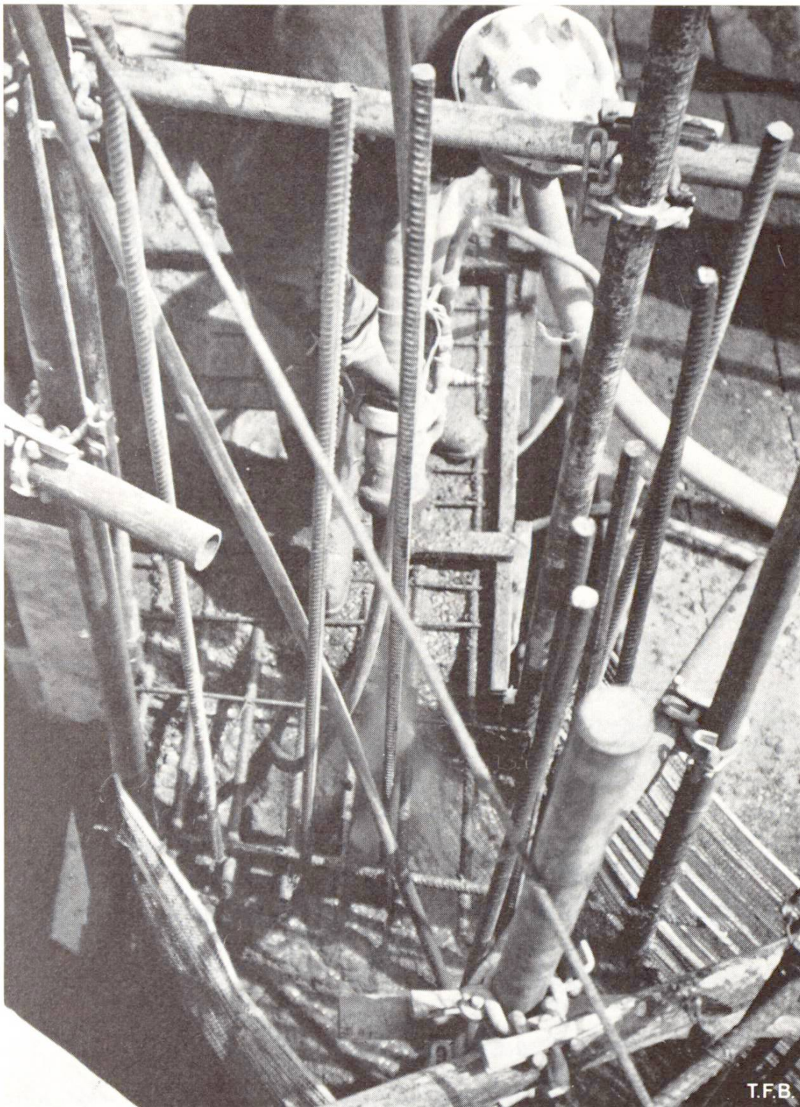
Abb. 1 Spritzbeton 0-15 mm, mit ca. 350 kg PC/m 3 , wird als Füllbeton ohne wesentliche Verluste in Streckmetall-Korb eingebracht. In einem zweiten Arbeitsgang werden die äusseren Seiten mit Spritzbeton 0-8 mm mit ca. 400 kg PC/m 3 abgedeckt (Turm der Kirche Abb. 4).
