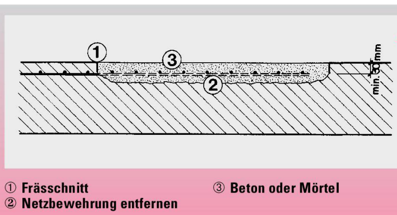
Abb. 3 Reparatur von Oberflächenschäden [5].
